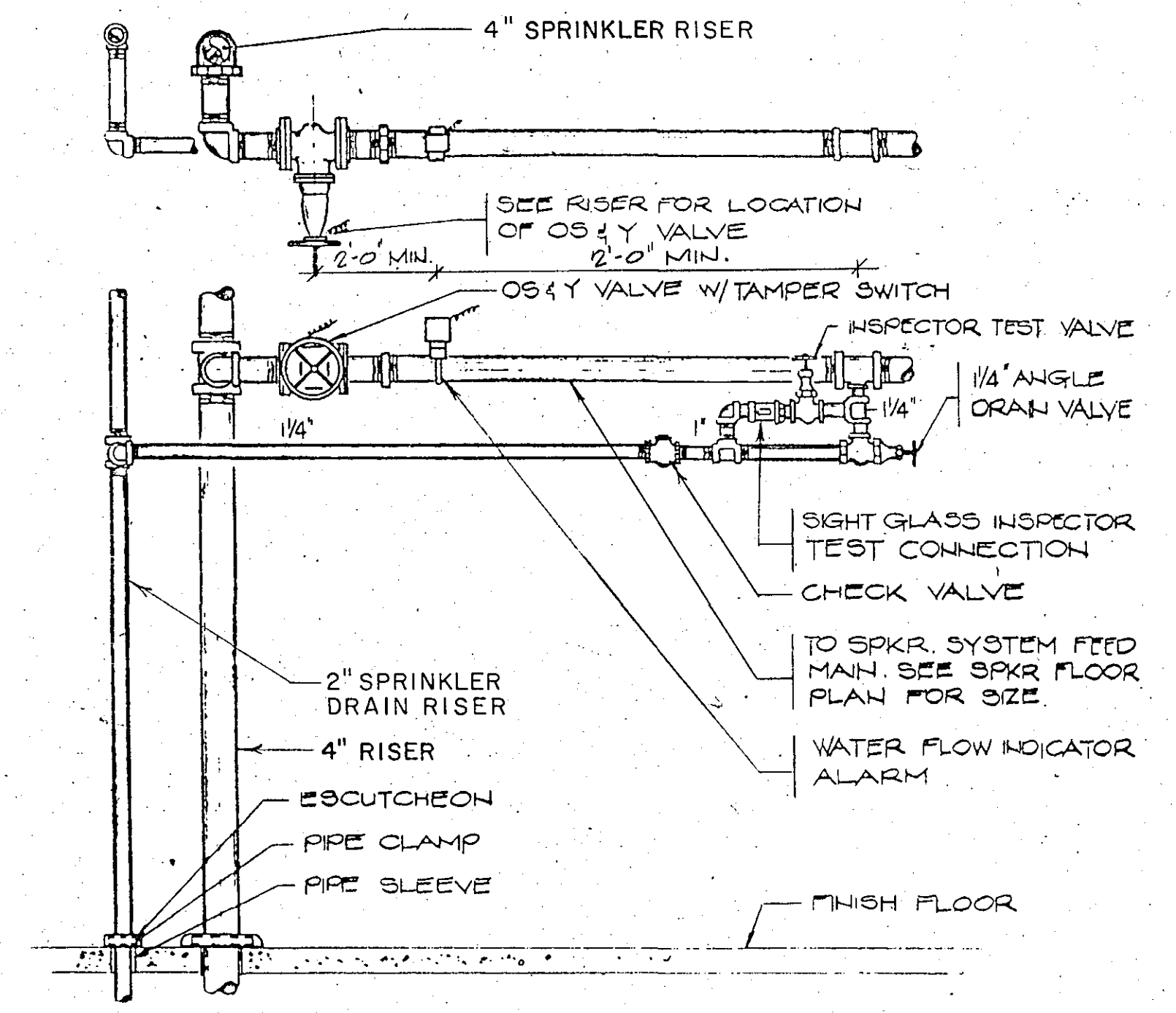
SPRINKLER RISER DETAIL N.T.S.
