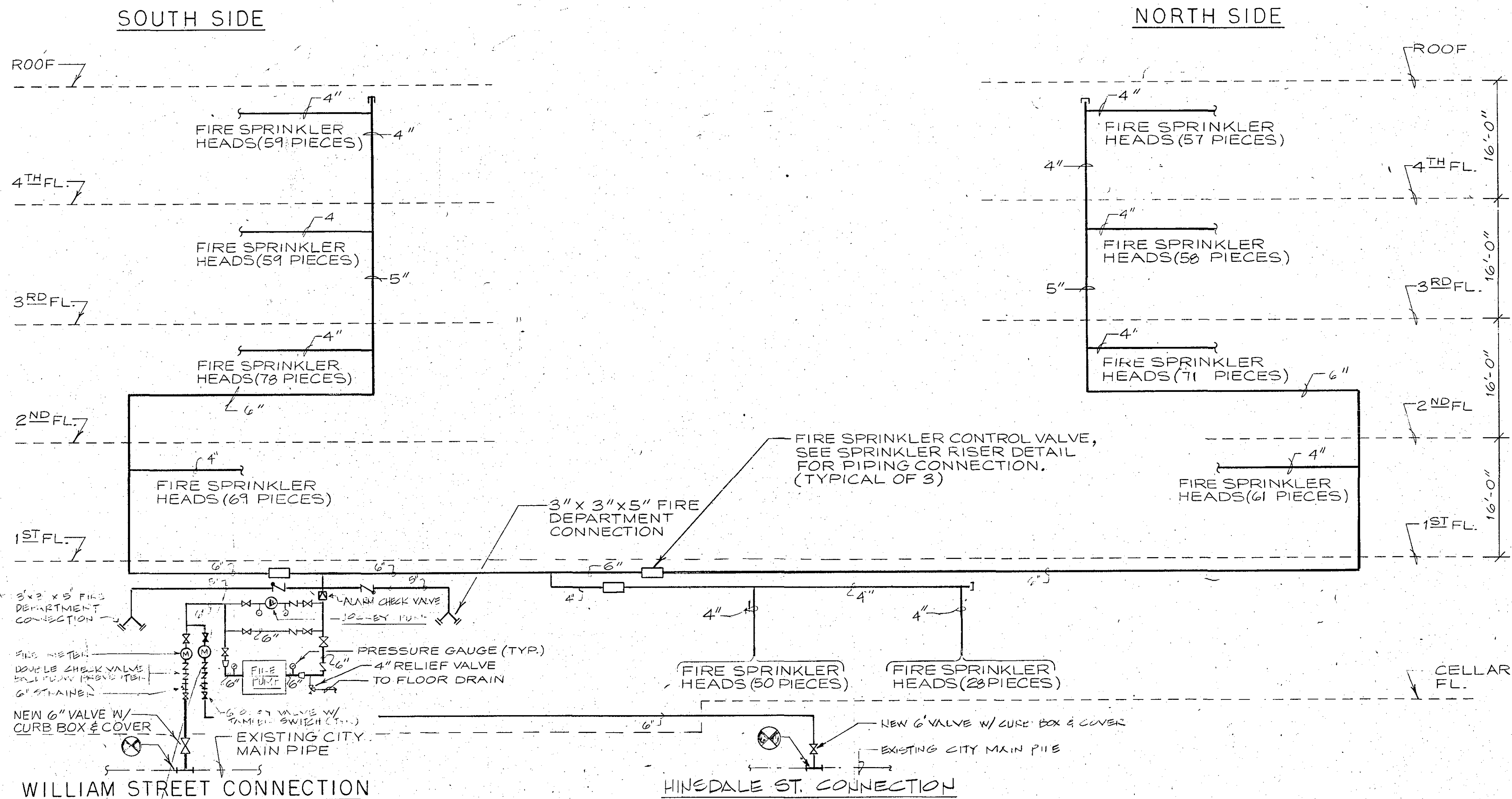
SPRINKLER SYSTEM RISER DIAGRAM N. T. S.
