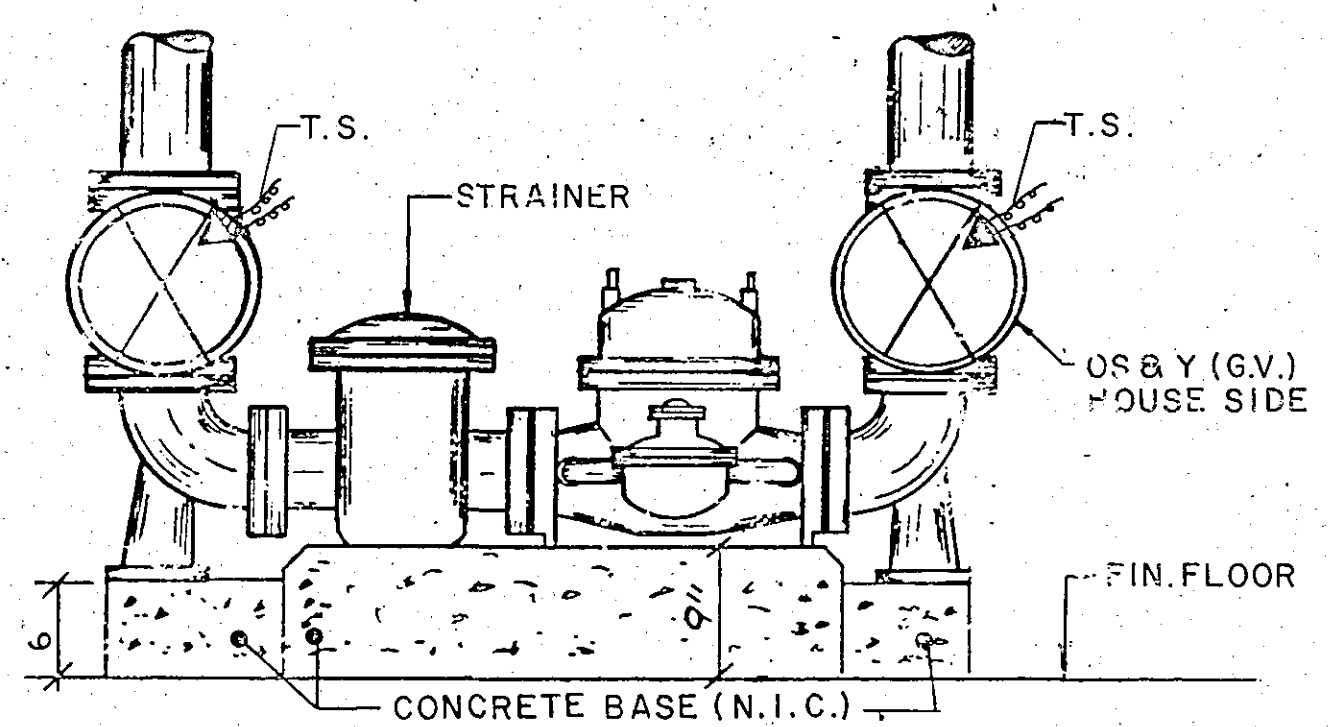
METER RIG SPRINKLER N. T. S.
